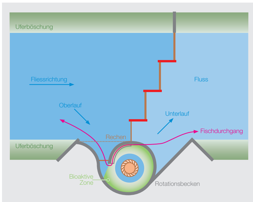
Bild 2 Grundriss eines GWVPP samt niedrigem Wehr.
