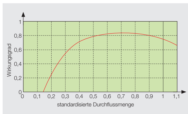
Bild 3 Wirkungsgradverlauf der Zotlöterer-Turbine im GWVPP.
